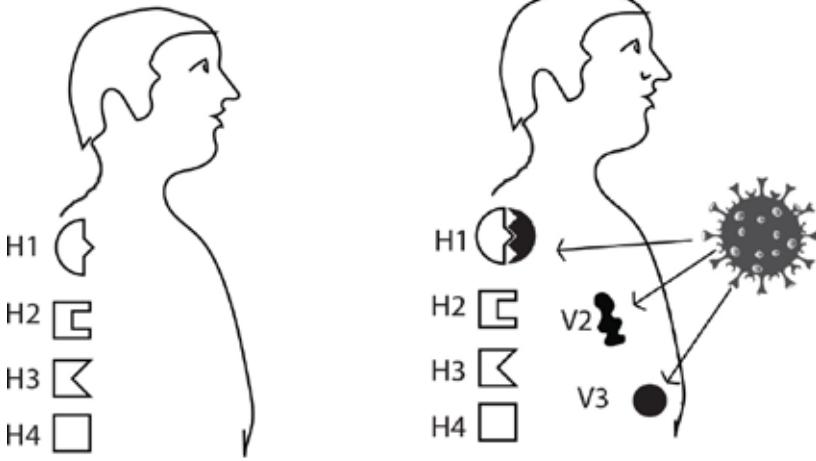
1. H1, H2, H3, H4 എന്നിവ മനുഷ്യകോശത്തിലെ സ്വതസിദ്ധമായ തന്മാത്രകൾ
