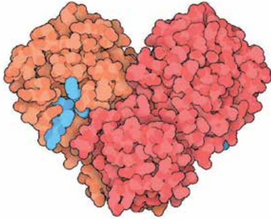
ചിത്രം 5: കൊറോണ വൈറസുമായി ബന്ധപ്പെട്ട ഒരു പ്രമുഖ തന്മാത്ര കമ്പ്യൂട്ടറിൽ ദൃശ്യവൽക്കരിച്ചിരിക്കുന്ന ചിത്രമാണ് ചുവടെ (SARS - Cov - 2 Main Protease) കേരള സർവകലാശാലയിൽ ലഭ്യമായ Discovery Studio Visualizer എന്ന സോഫ്റ്റ് വെയറിലാണ് ഈ ചിത്രം ദൃശ്യമാക്കിയിരിക്കുന്നത്.
