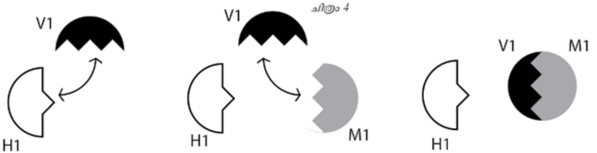
1. H1- V1 കൂട്ടചേർന്ന് H1 സ്വതന്ത്രമായി ശരീരത്തിന് ലഭ്യമാകാതെ ഇരിക്കുന്ന അവസ്ഥ അസുഖത്തിന് ഹേതുവാകുന്നു. 2. ഔഷധതന്മാത്ര M1 ശരീരത്തിൽ ലഭ്യമാകുന്നു. M1 ഉം V1 ഉം തമ്മിൽ മികച്ച ചേർച്ചയാണ് 3. V1 ഉം M1 ഉം തമ്മിൽ സംയുക്തം ഉണ്ടാകുന്നു. H1 അങ്ങനെ സ്വതന്ത്രമായി ലഭ്യമാകുന്നു.
